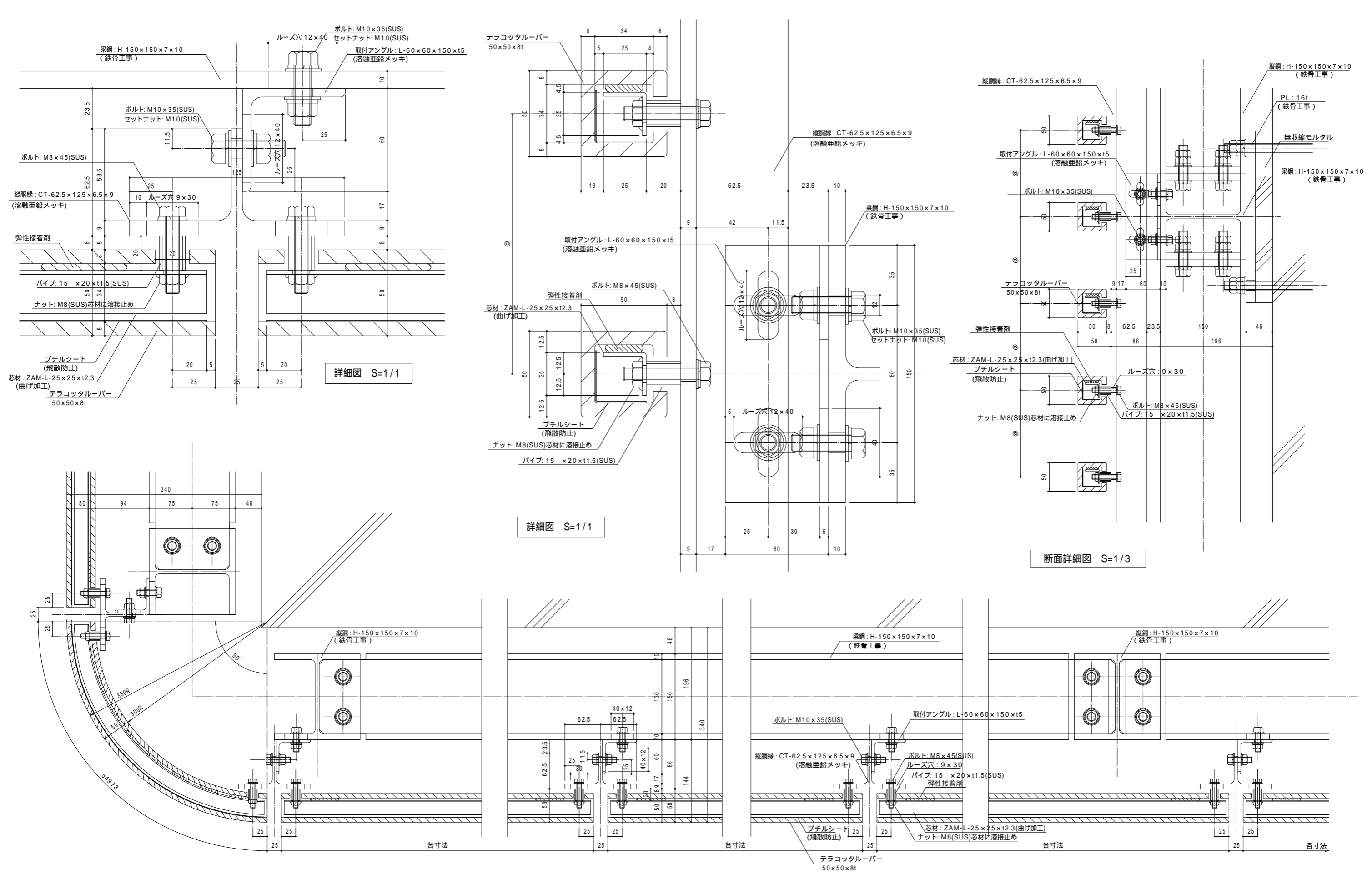
平面詳細図 S=1/3
